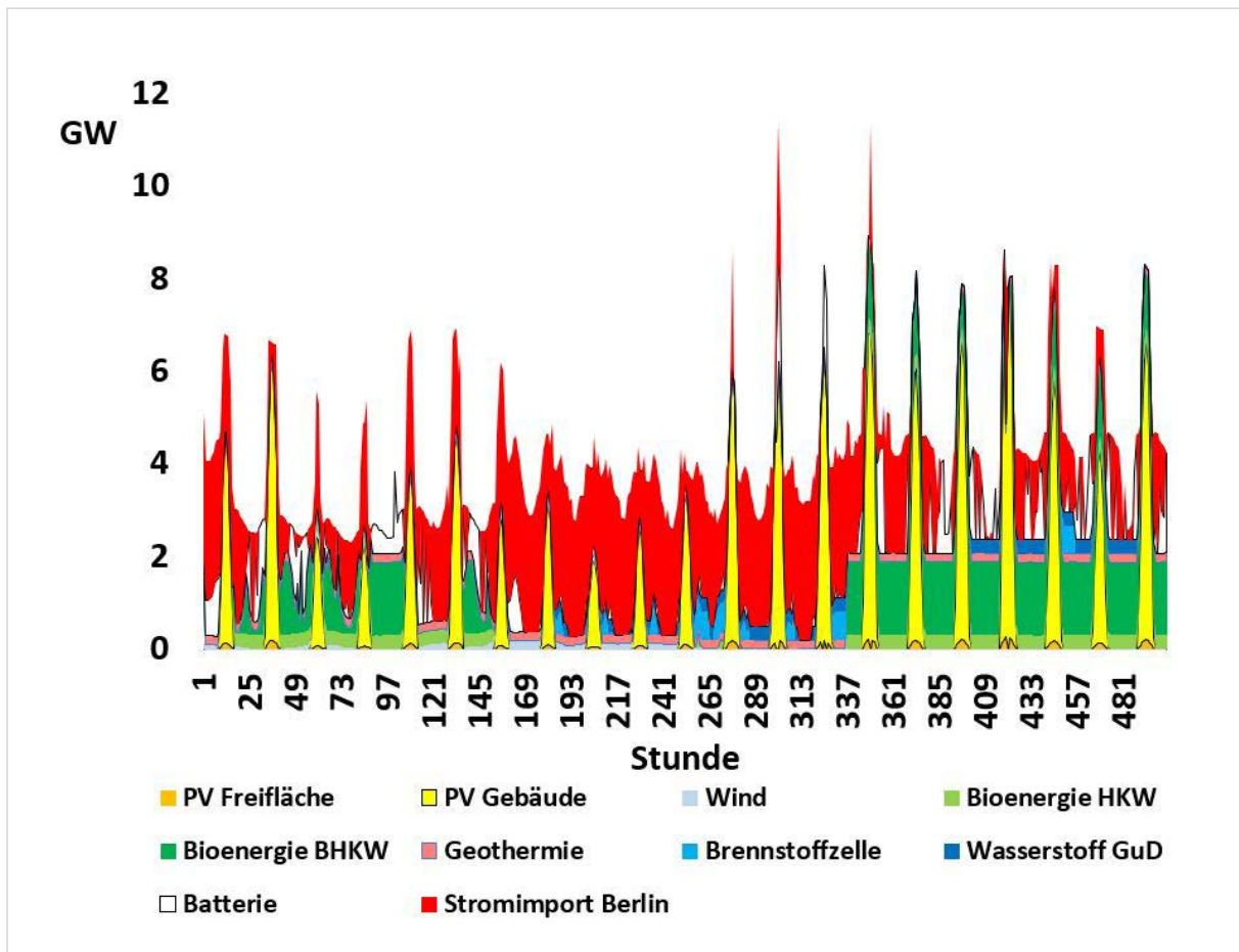
Abbildung 2: Stromerzeugung und Stromimport Berlins aus Brandenburg.
