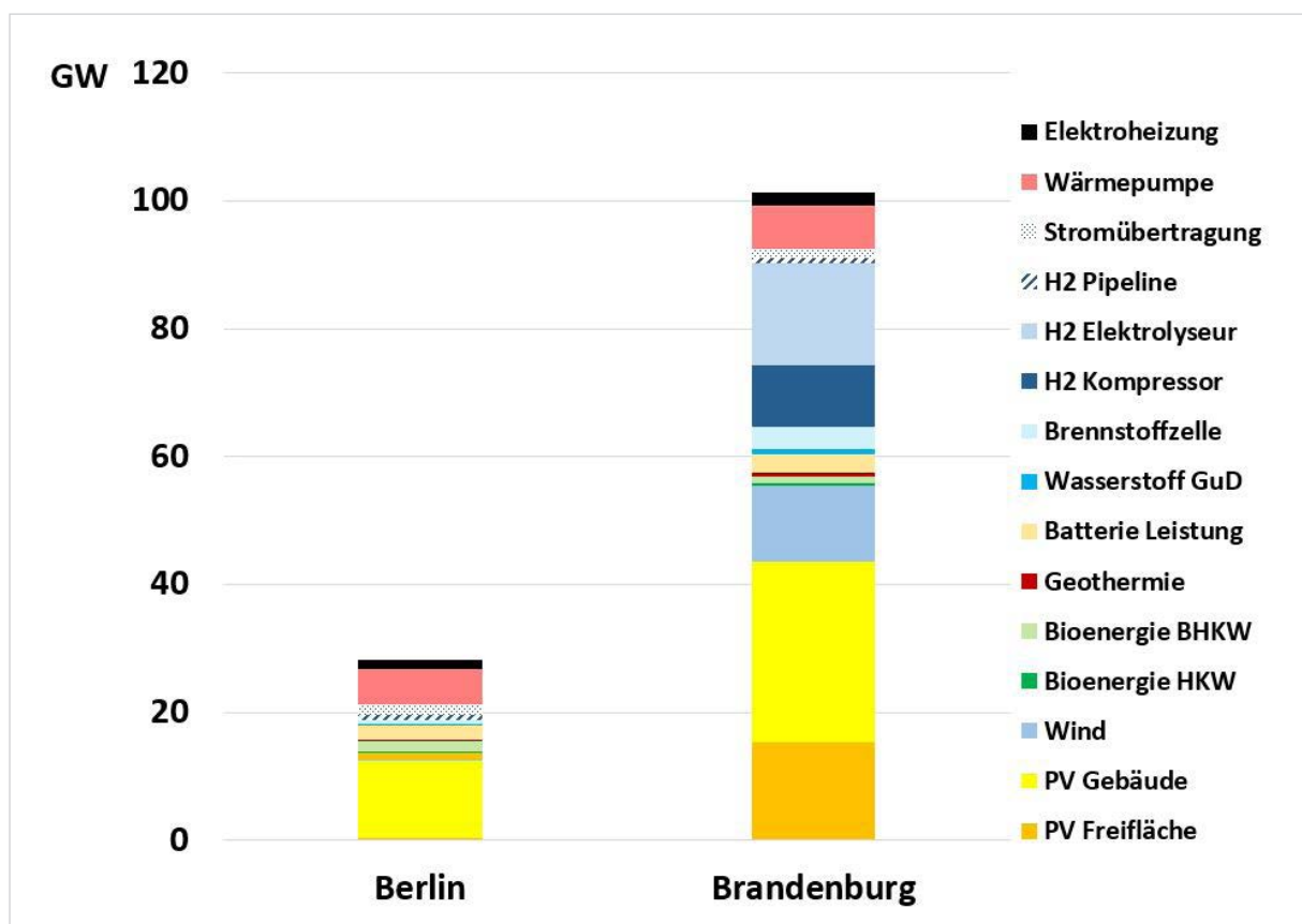
Abbildung 1: Erzeugungs- Umwandlungs- und Energieübertragungskapazitäten für eine 100% Vollversorgung aller Energiesektoren auf Grundlage erneuerbarer Energien im EWG-Szenario.
