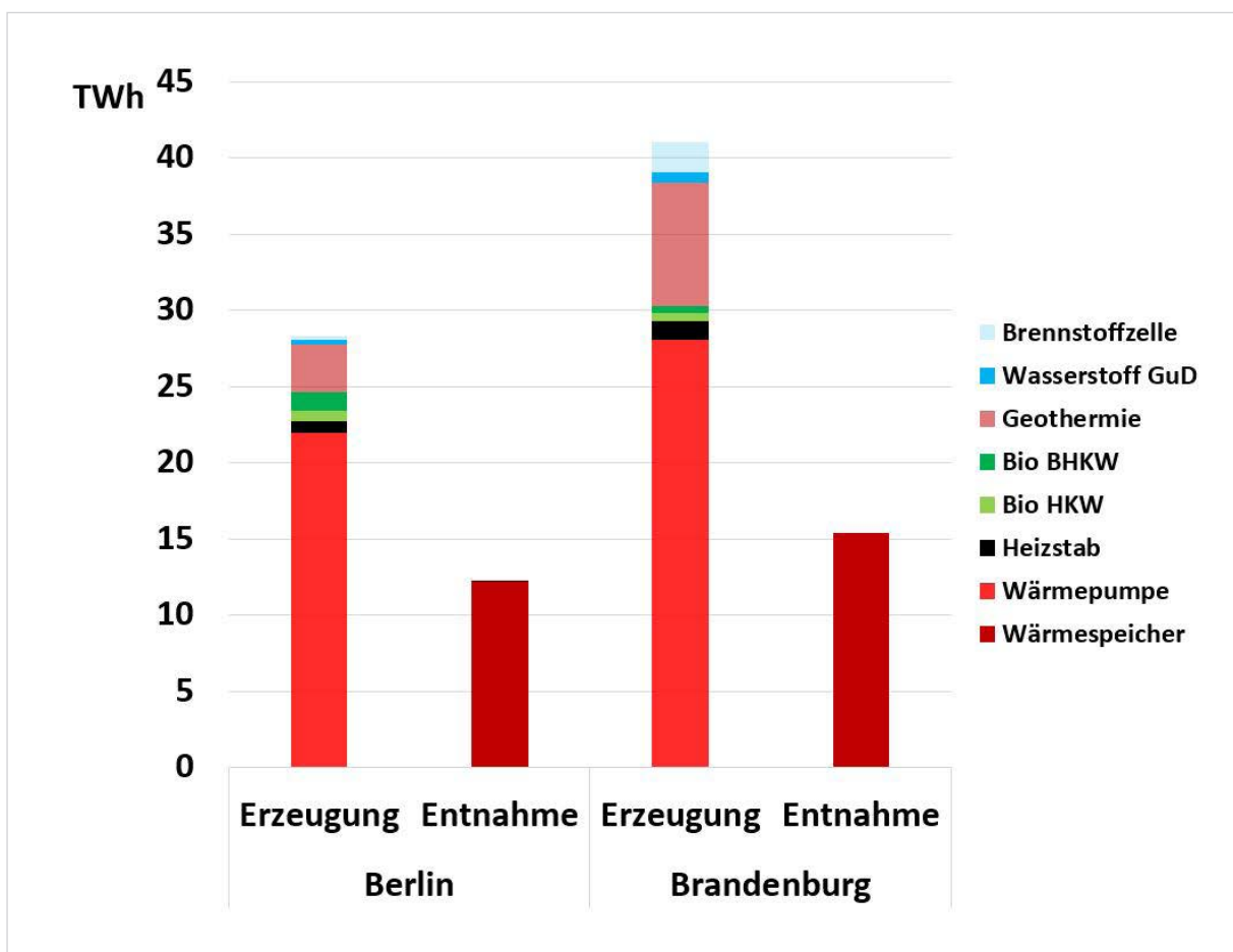
Abbildung 5: Wärmeversorgung in Berlin und Brandenburg im EWG Szenario. Wärmepumpen dominieren den optimalen EWG Erzeugungsmix, der im jeweils unteren Teil der Balken dargestellt ist.
